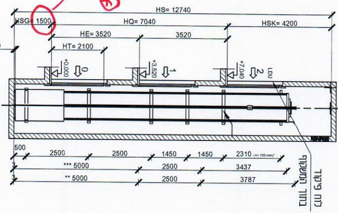
Section A-A 1:100
